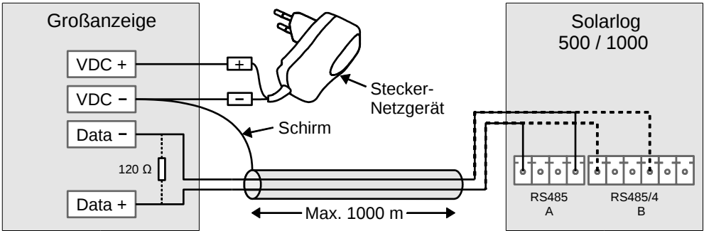
Abbildung5.10: Anschluss-Schema, SolarLog
