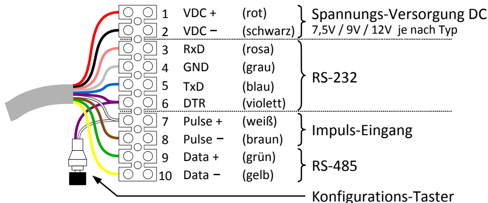
Abbildung4.1: Anschlussbelegung, Lüsterklemmen
