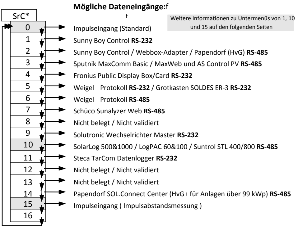
Abbildung6.2: Konfigurationsmenü
