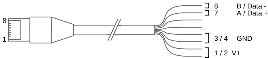
Abbildung5.6: Kabelbelegung, Sputnik CAT5 Netzwerkkabel
