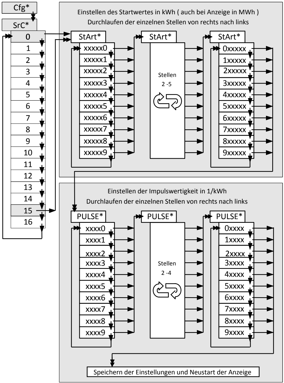
Abbildung6.3: Konfigurationsmenü, Unterebene Impulseingang
