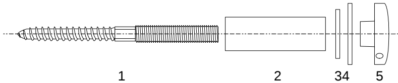
Abbildung3.2: Befestigungsmaterial, Glasanzeigen
