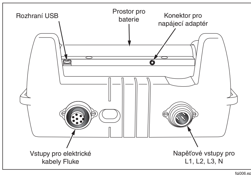
Obrázek 3. Konektory přístroje Power Logger
