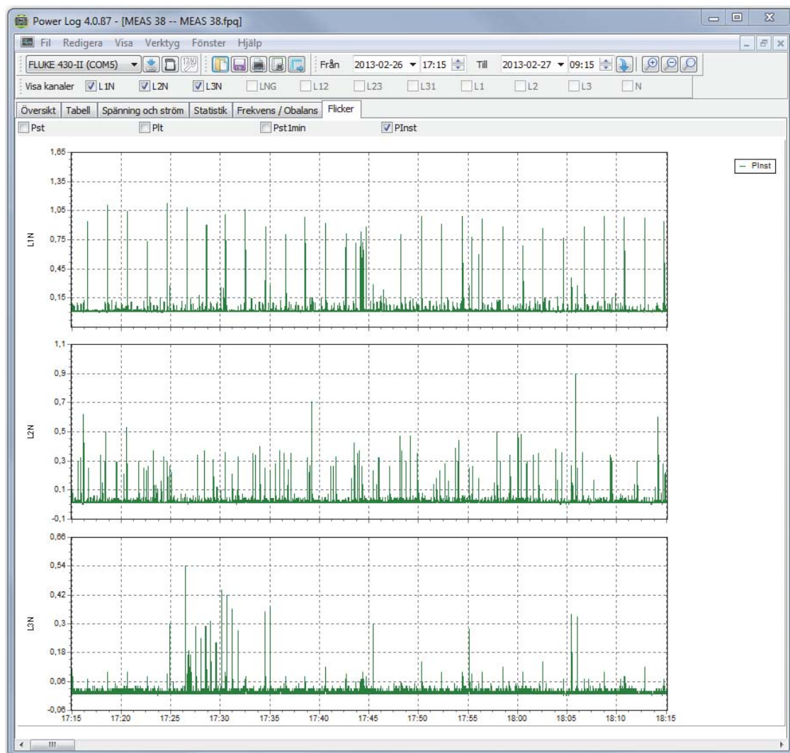
Figur 13. Flicker-vågformer
