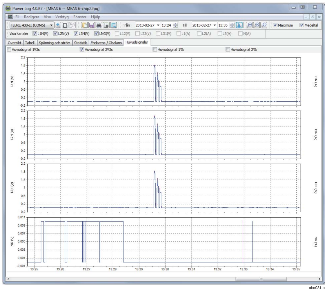
Figur 18. Vågformer i Huvudsignaler
